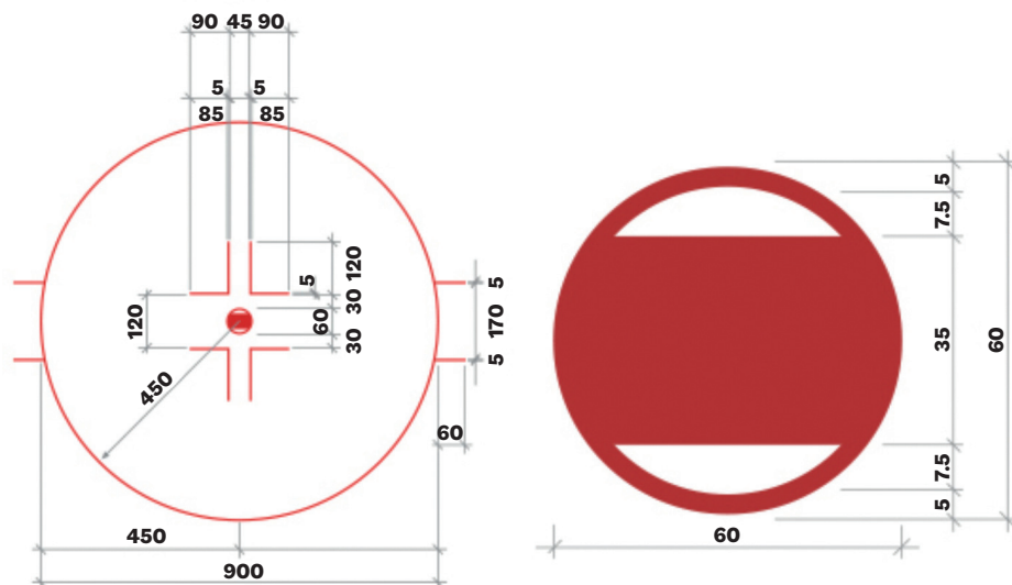
FIGUR 2 – TEKNINGSCIRKEL & TEKNINGSPUNKT
