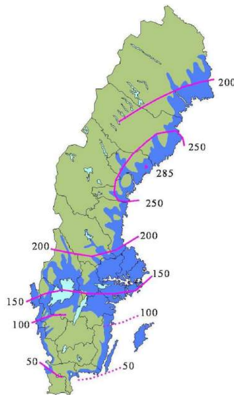
Figur 18 Det mörkblå på kartan visar områden som idag utgörs av land, men som efter den senaste istiden låg under vatten. Siffrorna anger högsta kustlinjens höjd över dagens havsyta angivet i meter. Karta hämtad från SGU-rapport 2019:15.
