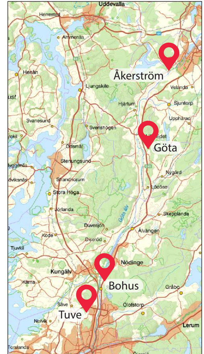
Figur 28 Göta älv har vid flera tillfällen drabbats av jordskred, varav de allvarligaste är utmärkta på kartan.
