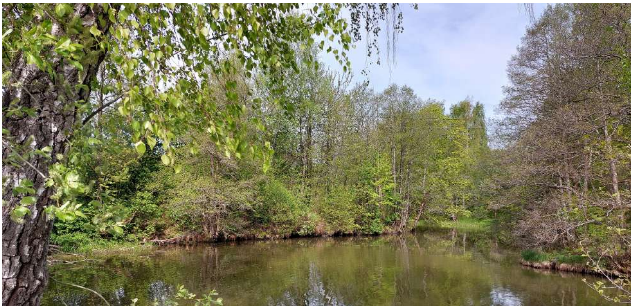
Figur 211 Strömsbäcken är ett betydelsefullt habitat för fågel.
